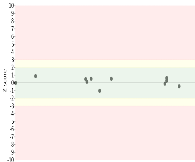
Gráfica 22 Z-score
