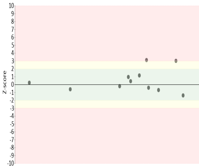
Gráfica 10 Z-score
