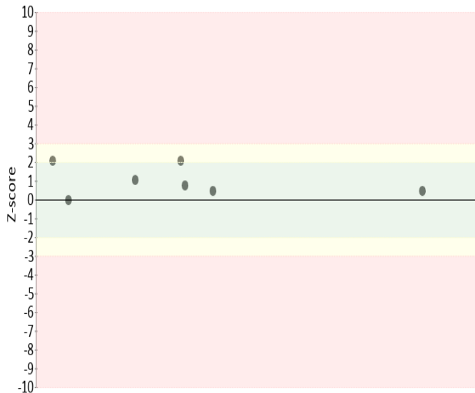
Gráfica 4 Z-score
