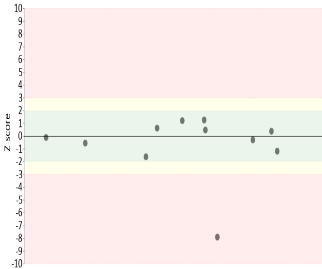
Gráfica 16 Z-score
