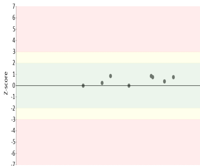
Gráfica 19 Z-score
