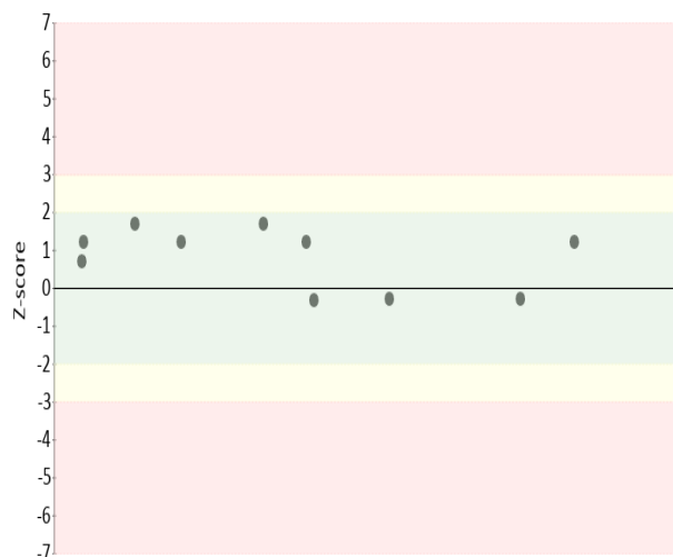
Gráfica 7 Z-score
