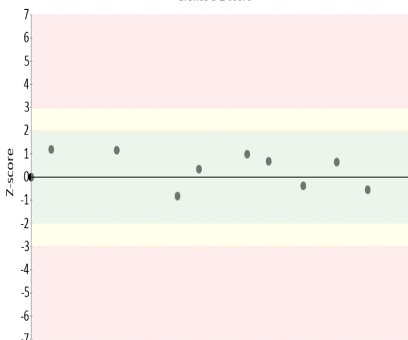
Gráfica 3 Z-score
