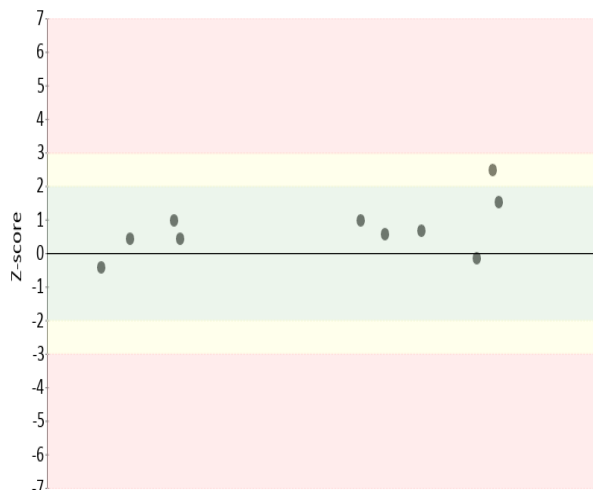
Gráfica 13 Z-score
