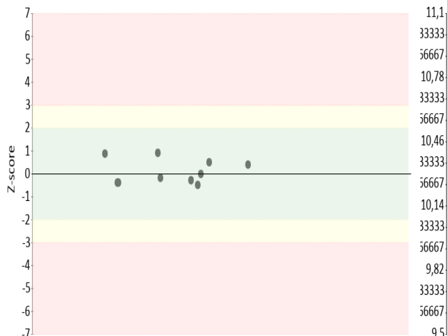
Gráfica 19 Z-score
