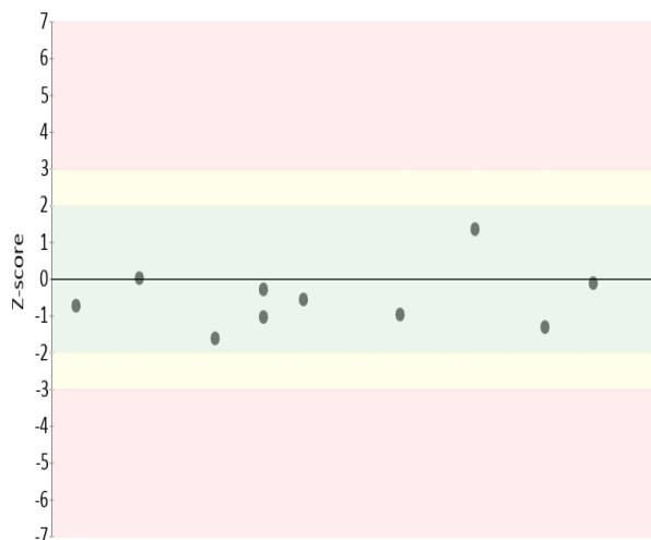
Gráfica 15 Z-score
