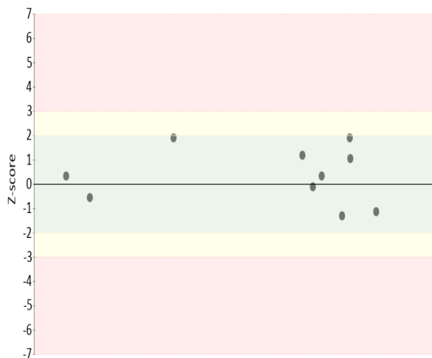
Gráfica 9 Z-score
